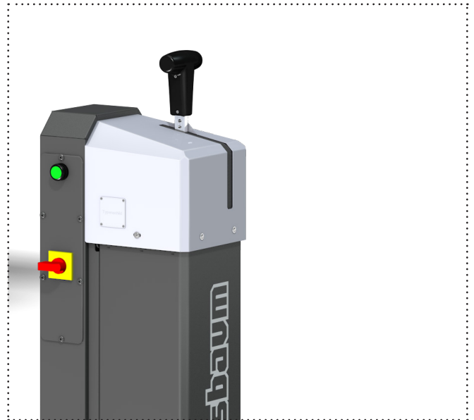
La leva di comando NUSSBAUM permette il controllo della velocità di discesa. The NUSSBAUM Commander offers variable lowering speeds.
